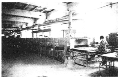
油烧辊道窑生产线
