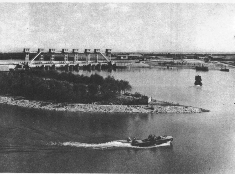
汉北水利工程一瞥。
