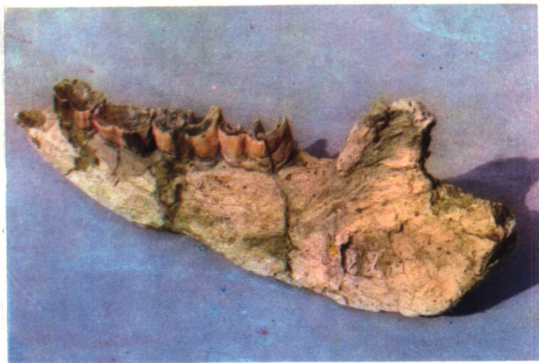
从黑隅里出土的二十九种动物遗骨之一——大双角犀牛化石。
