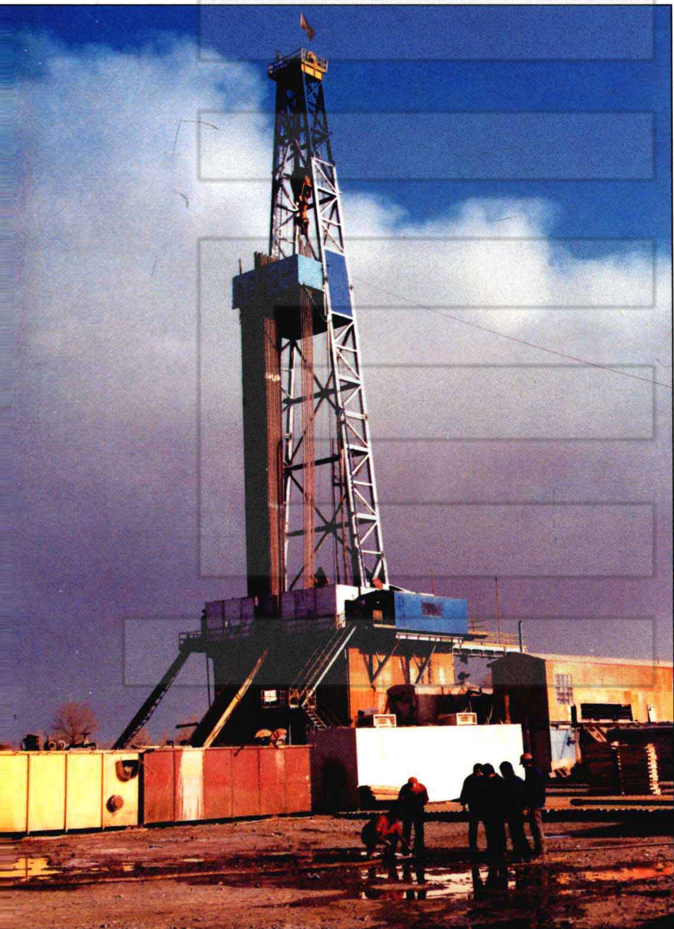
電動 900 米深井鑽機
