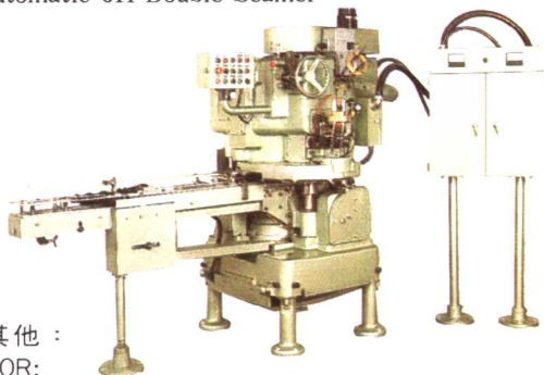
S-B45 6H 自動封罐機 Automatic 6H Double Seamer
