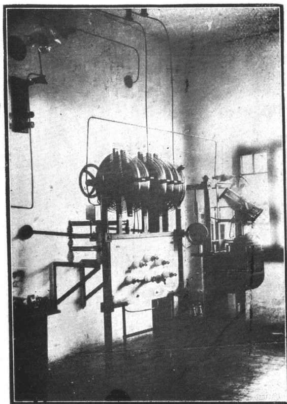
吳淞電台五千瓦特火花式發報機
