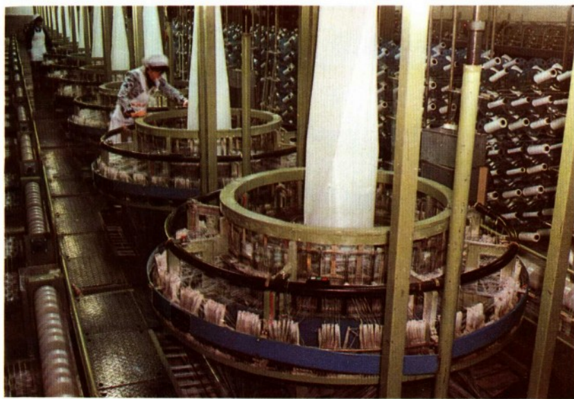
永红乡永红塑料编织厂四梭圆筒织机车间
