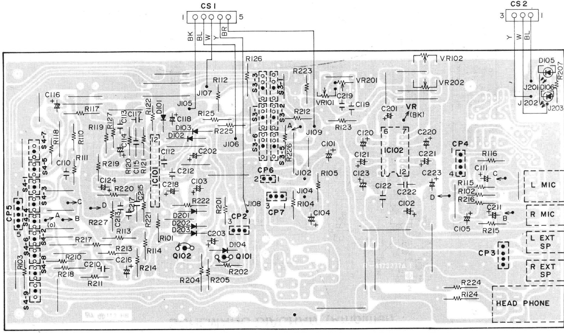
POWER P.C.B. Bottom
