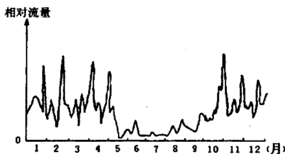
图2 某河相对流量过程曲线示意图
