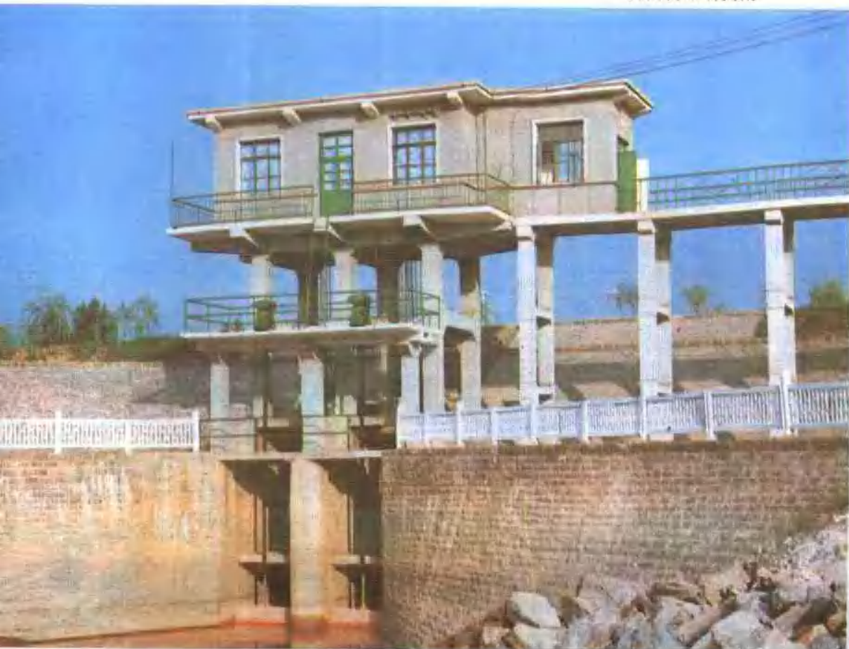
济南杨庄引黄闸
