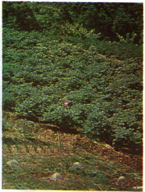
牡丹
