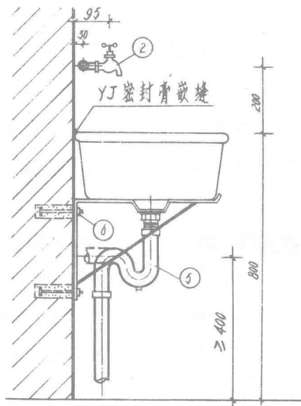
侧面图
