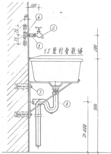
侧面图
