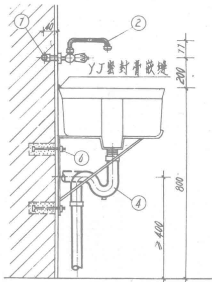
侧面图
