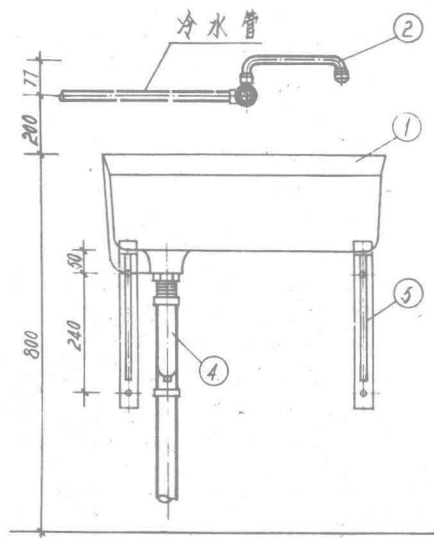
立面图
