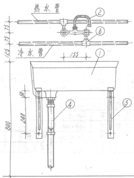
立面图
