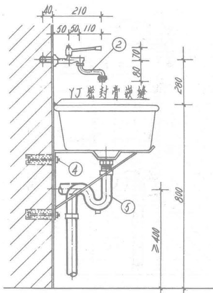
侧面图
