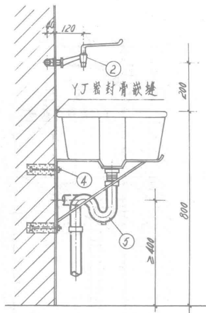
侧面图
