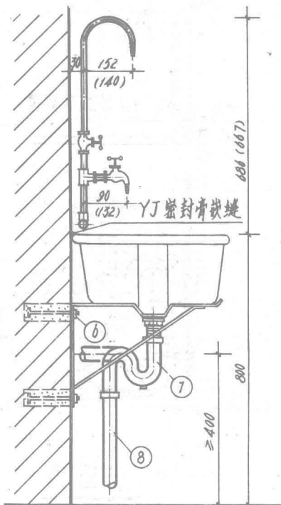
侧面图
