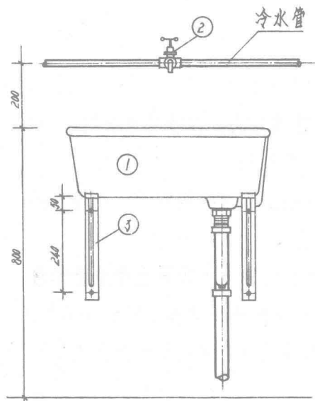
立面图
