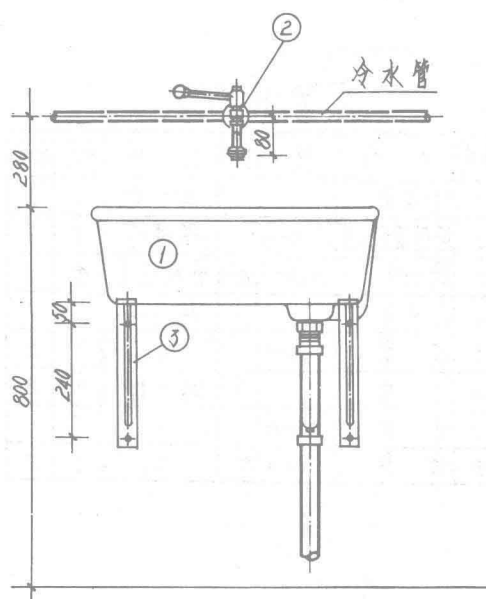
立面图
