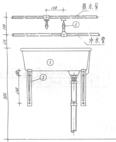
立面图
