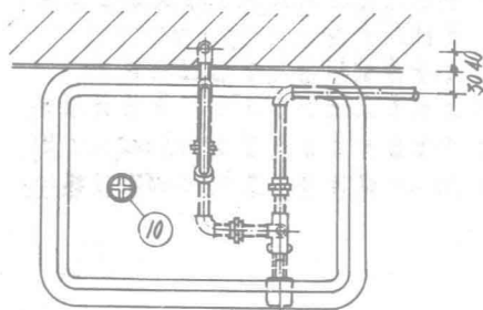
平面图
