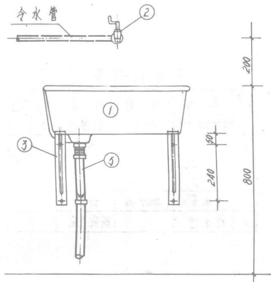
立面图
