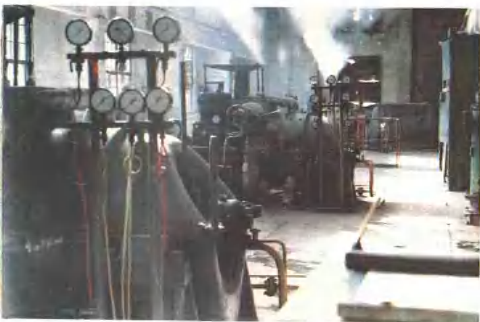
← 正常运行的汽轮机
