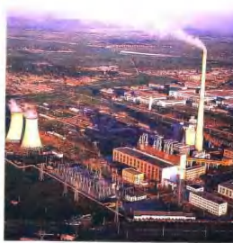
新近口电厂—装机容量145MW，年发电量400万度。为唐山市最早建设的热电厂
