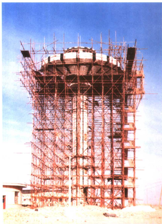
泽普石化厂伞型水塔
