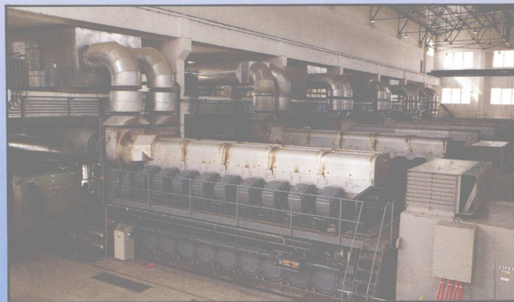
▲ 新建成投產的生明發電廠6.5萬千瓦發電機組
