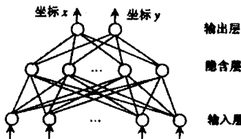
图 2 用于监测截面温度场中心的神经网络模型 Fig. 2 Neural network model
