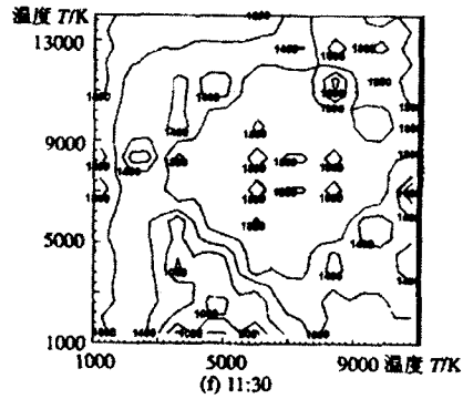
图 1 负荷变化过程中不同时刻的截面温度场 Fig. 1 Section plane temperature field at different points of the process
