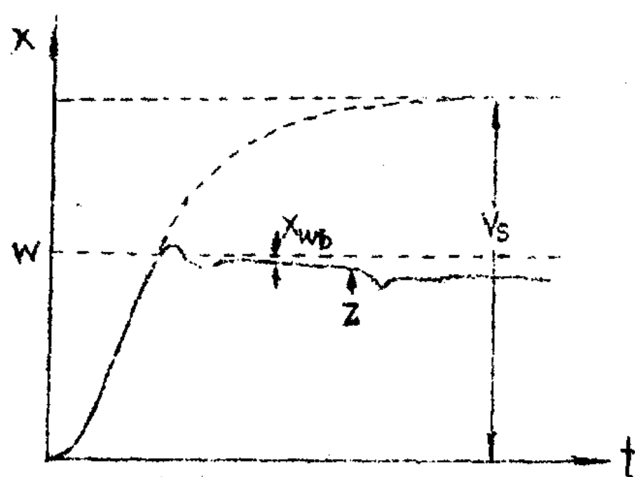
图11 PD-调节器·启动过 程和干扰Z
