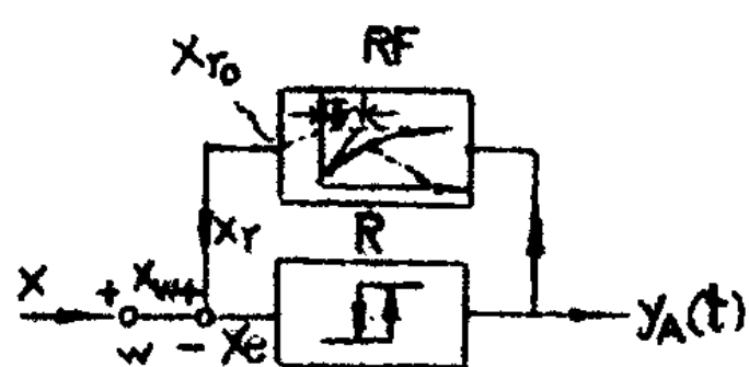
图7 具有滞后反馈作用的两点调节器PD调节器; 具有滞后再调(虚线)反馈作用的PID调节器。
