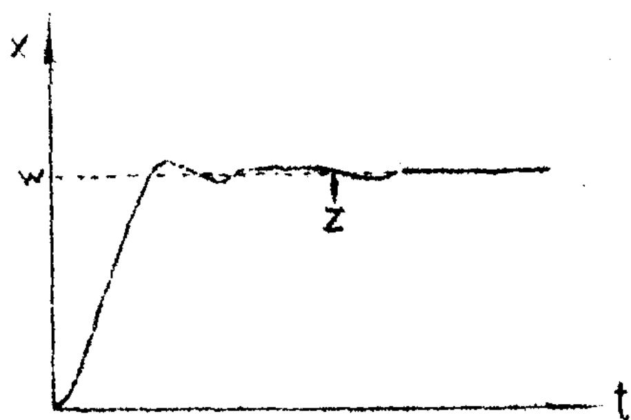
图 1 2 PID-调节器、 启动过程和干扰 Z
