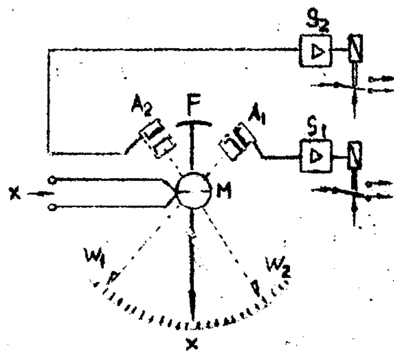
图 1 4 带有感应抽头装置的测量机构调节器
