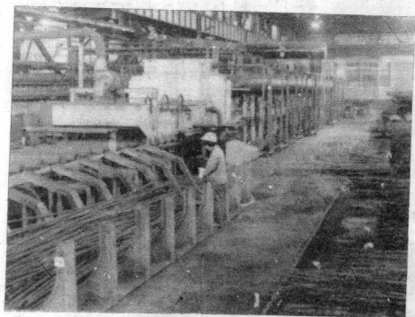
◁自行设计制造的采用微机控制的辊底式连续退火炉。
