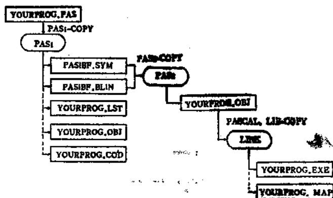
图 2.1 如何翻译你的程序
