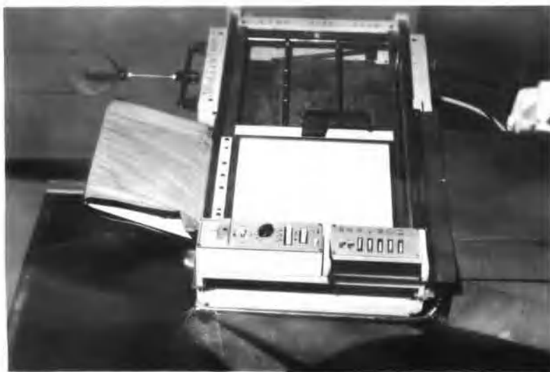
3000毫安X光机
