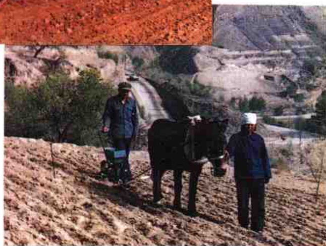
BFX—1 型水平沟施肥播种机播种
