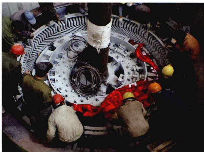
安装发电机转子
