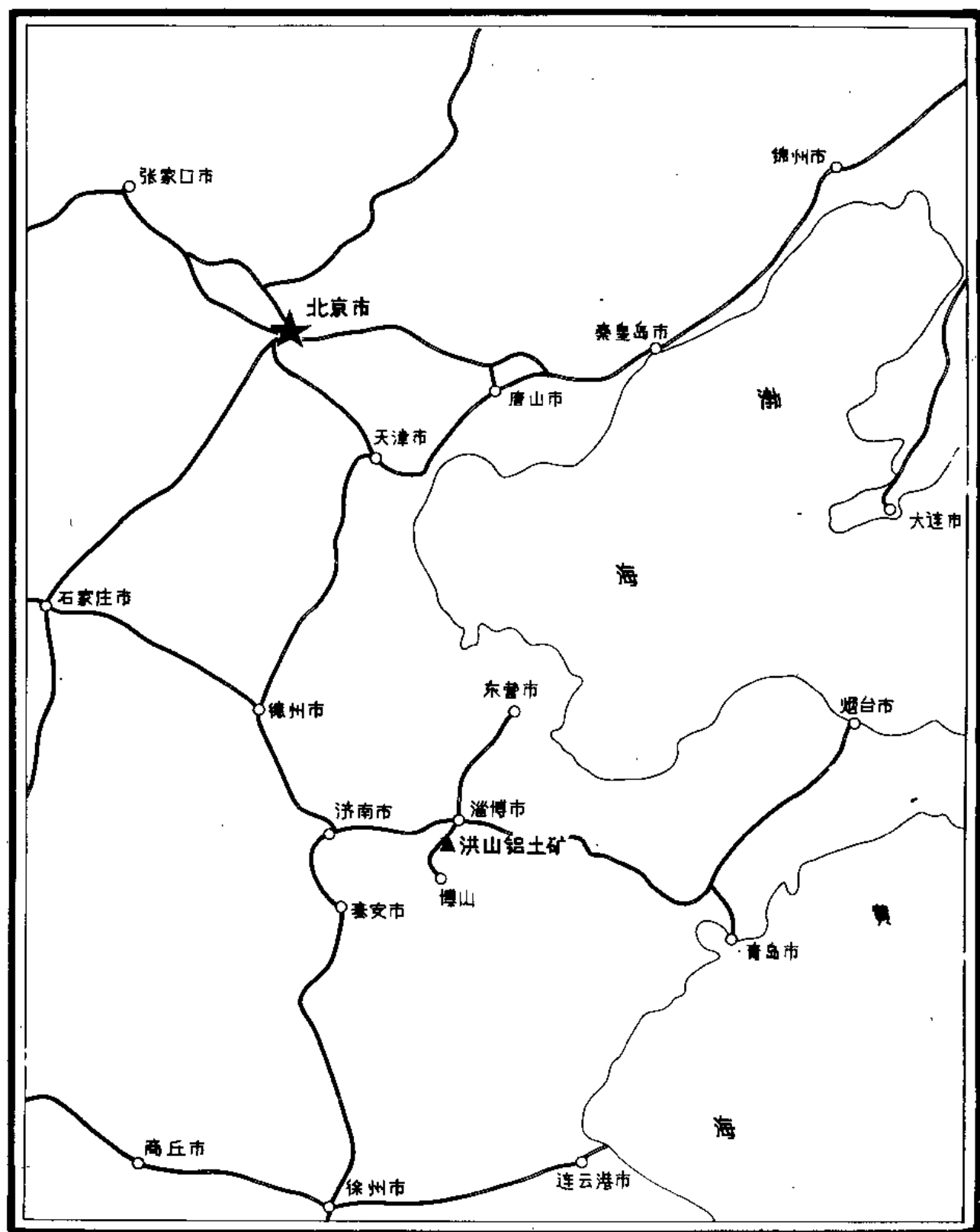
洪山铝土矿交通位置图
