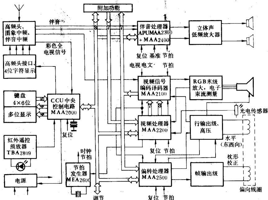
图 5 DIGIVISION 2000型数字电视机方框图
