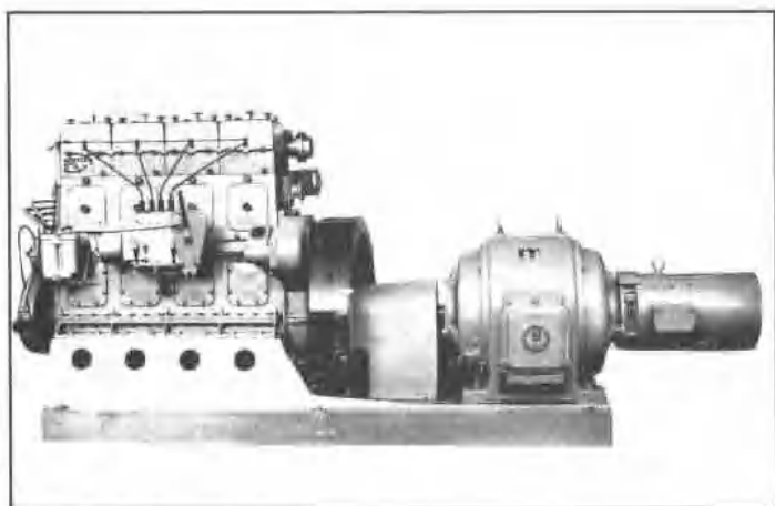
50 年代产品 4160 柴油发电机组
