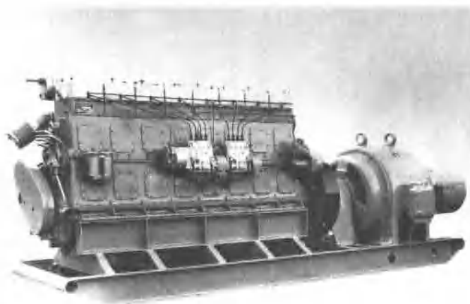
50 年代产品 8160 柴油发电机组
