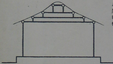
九架無廊
