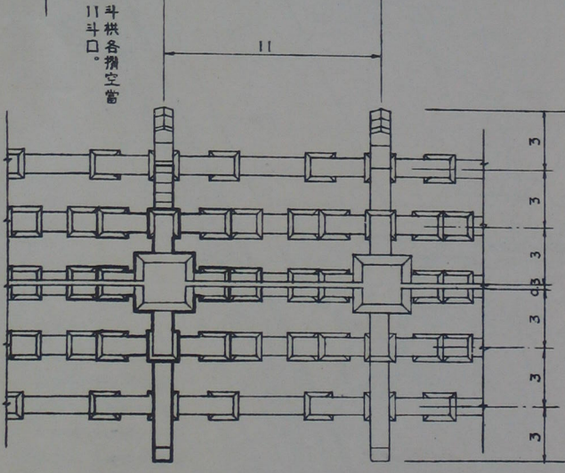
平身斗拱
