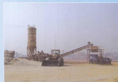
■ 松山湖大道水泥稳定土拌和站
