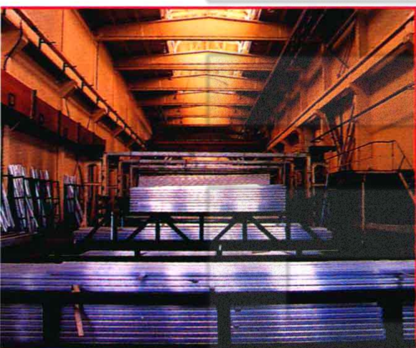
鋁型材氧化着色生產線
