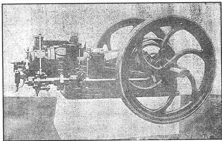
▲ 华丰机器厂生产的柴油发动机（区档案馆提供）
