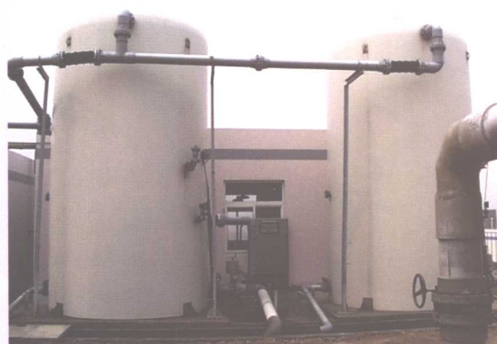
压力过滤罐
