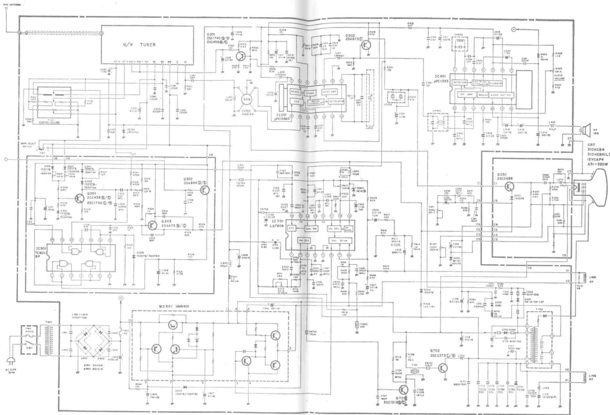
10. 日立M1201 12英寸电视机电原理图 (4—26页图1(a))
