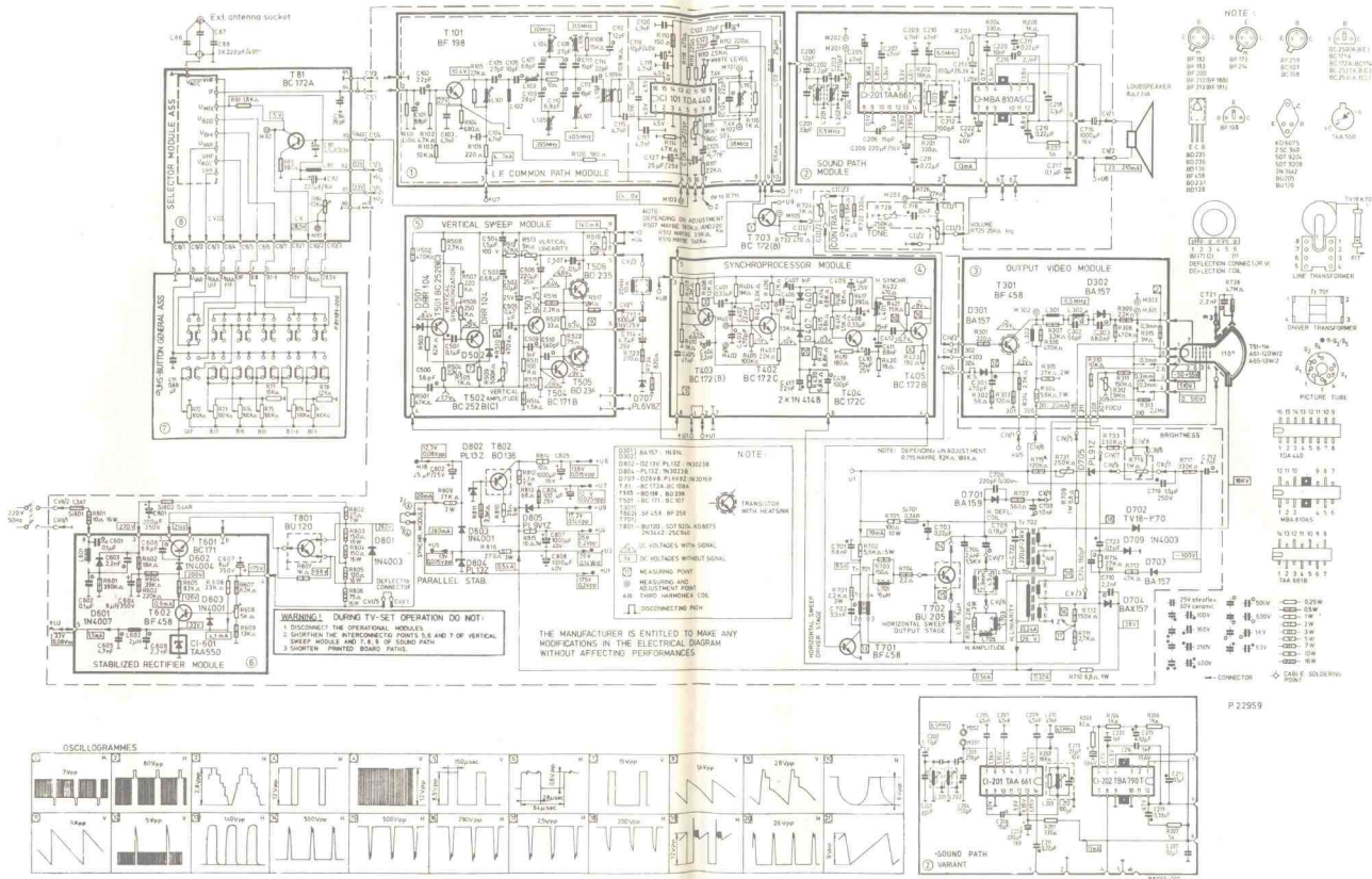
2. 罗马尼亚 244 型黑白电视机电原理图 (1—28 页)
