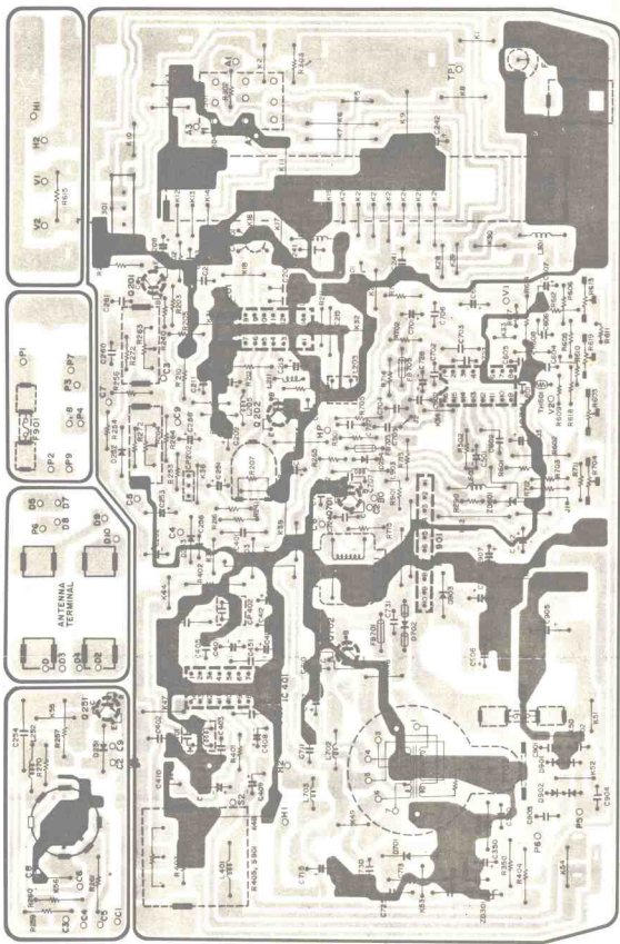
10. 日立M1201 12英寸电视机印刷电路板 (4—26页图(b))
