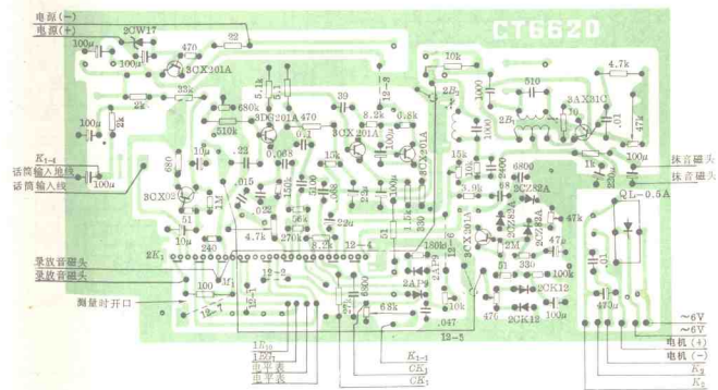
11. 美多牌CT6620型台式收录音机印刷电路板 (一)
