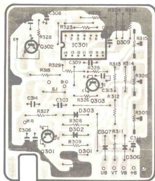
10. 日立M1201 12英寸电视机印刷电路板 (4—26页图(c))
