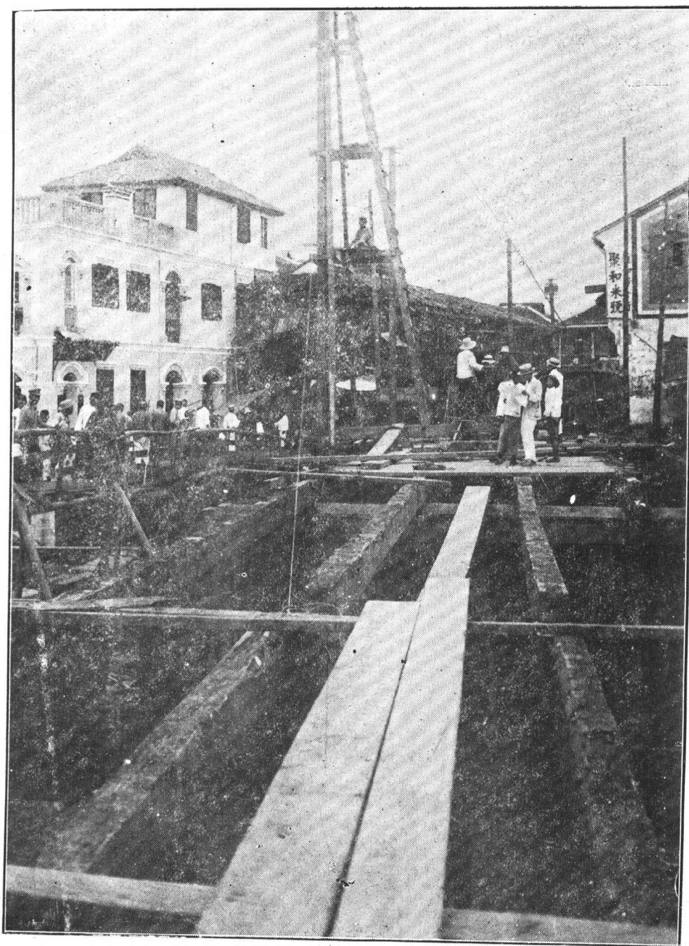
修 理 下 關 龍 江 橋 之 施 工 情 形
