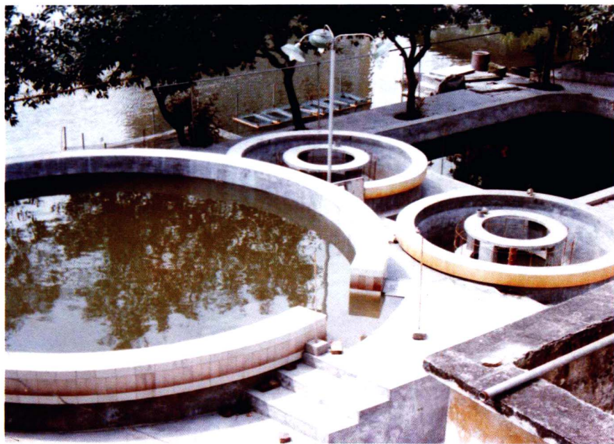
■ 标准产卵池和孵化环道设施
