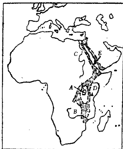
图 1-10 东非裂谷带示意图
