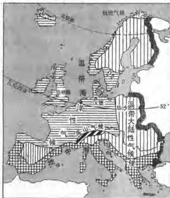
图1-2 欧洲西部气候类型图
