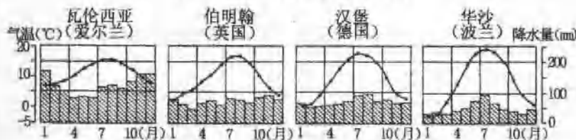
图1-3 欧洲西部四地各月气温与降水量分配图
