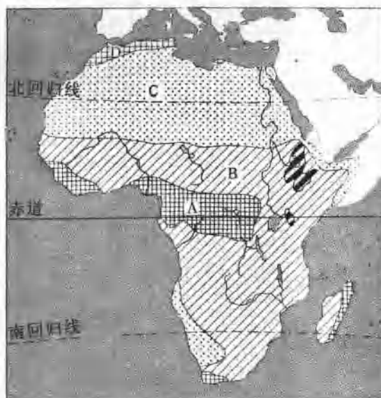
图 1-9 非洲气候分布图
