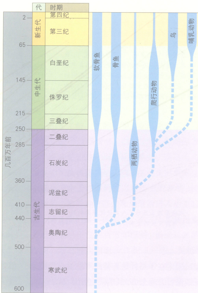
此表说明动物从原生代第一期到新生代的变化。
