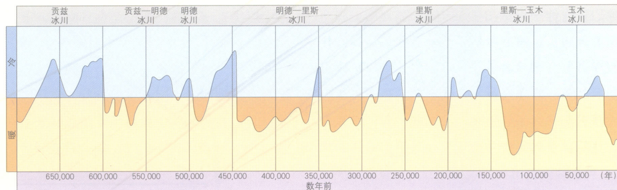
图表表明地球上经历的主要冰期和间冰期。
