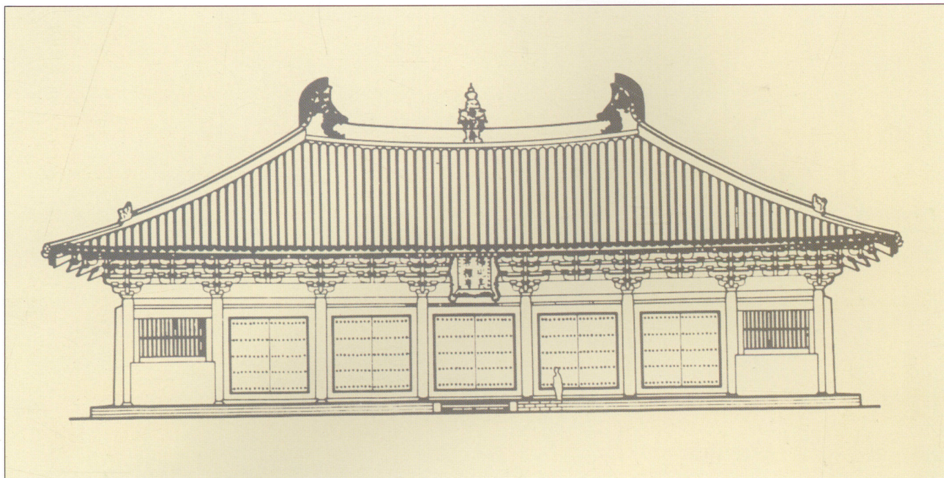
▲ 佛光寺东大殿正立面图
