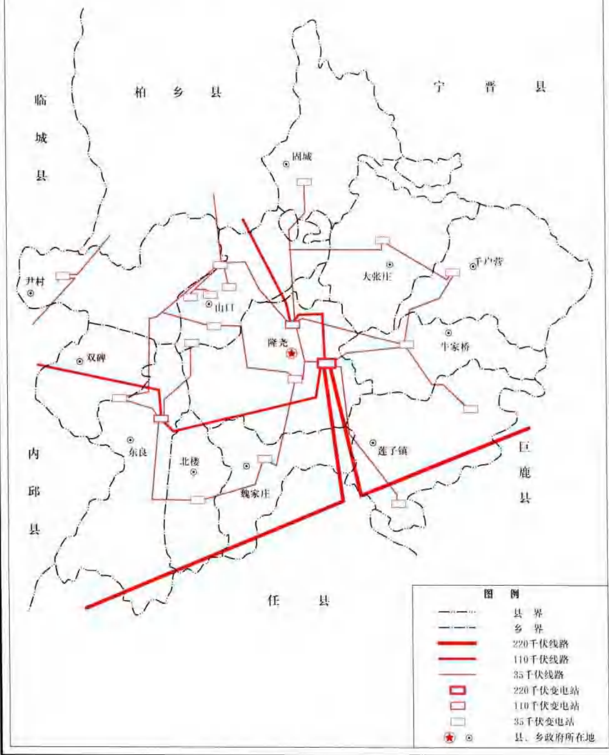
隆尧县2000年电网现状图
