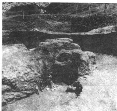
7. 一九七九年在铜录山十一号矿体冶炼遗址出土的春秋早期炼铜鼓风竖炉(残体)。 (潘红耘摄影)
