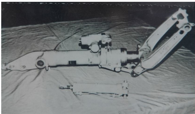
1969~1977 年学校改为国营长征机械厂期间生产的飞机起落架
