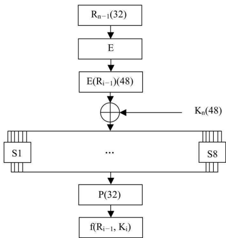
图 1.7 f(R, K) 函数的计算
