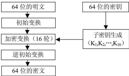
图 1.4 DES 数据加密基本流程
