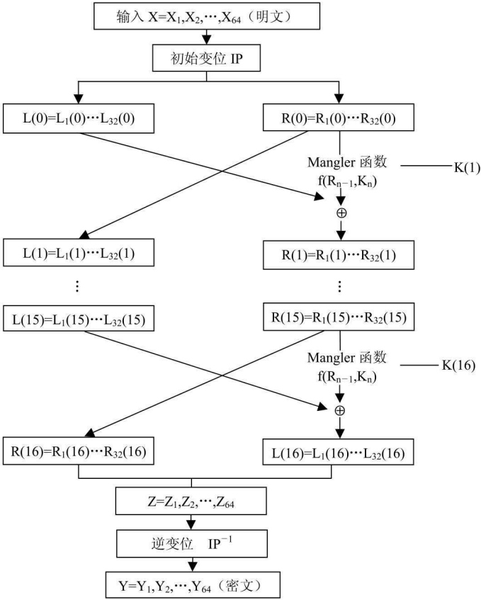
图 1.5 RES 算法框图（数据部分）
