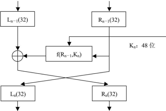
图 1.6 第 n 轮的加密变换
