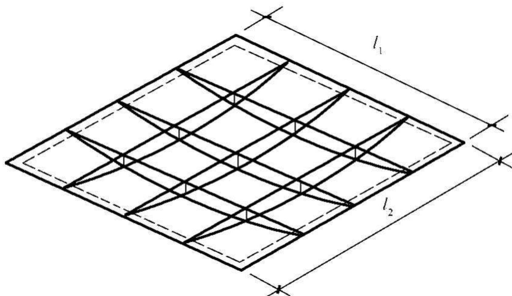
图 2-3 双向板
