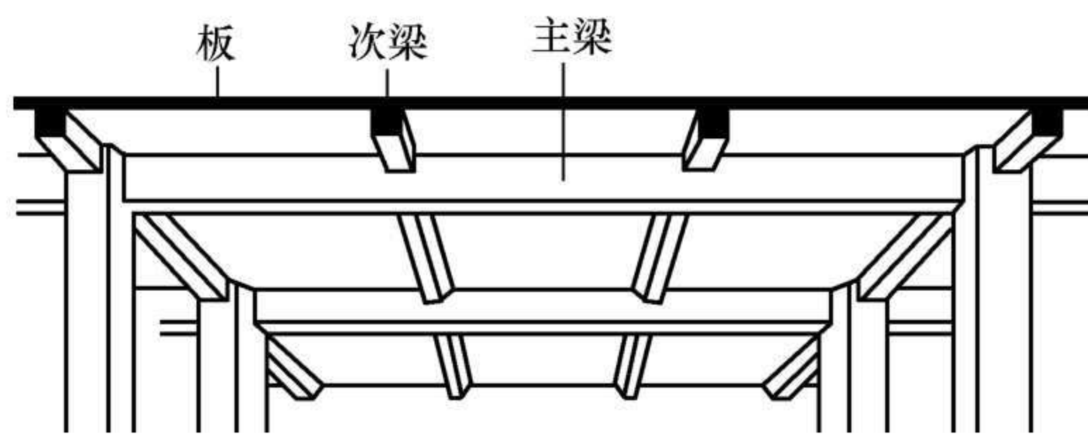
图 2-1 现浇钢筋混凝土肋形楼盖
