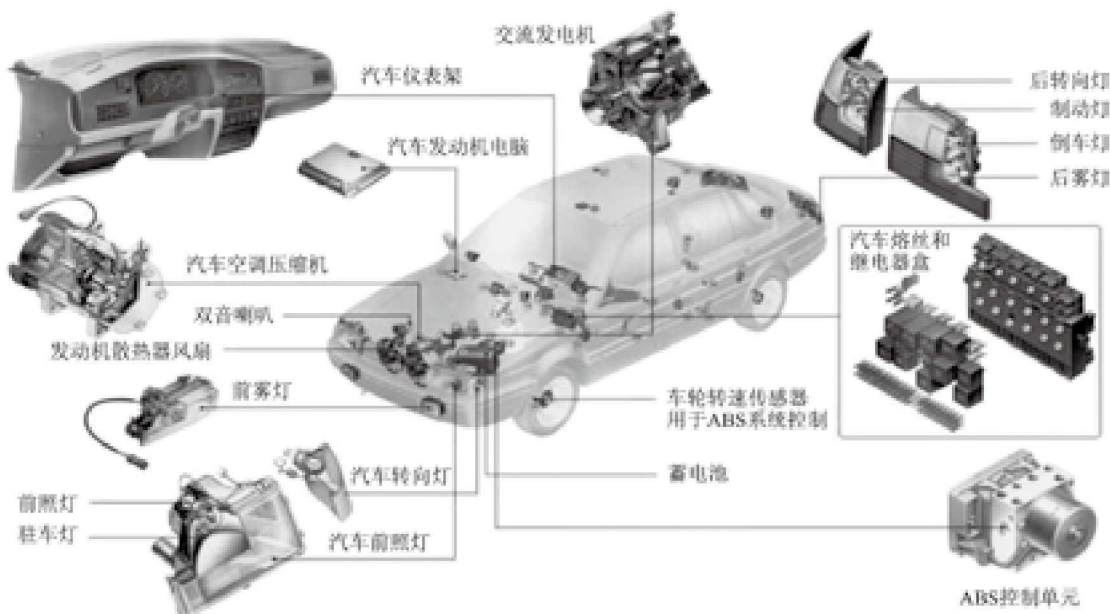
图 1-1 汽车电器分布与组成
