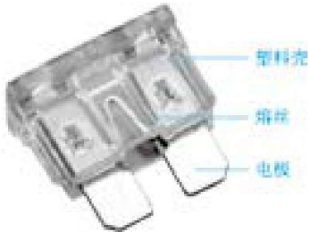
图 1-4 插片式熔断器的组成
