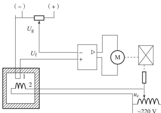
图 1-3 炉温闭环控制系统
