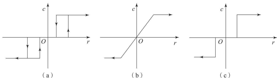
图 1-7 典型非线性环节特性
