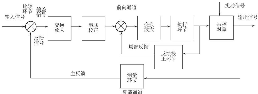
图 1-6 闭环控制系统方框图
