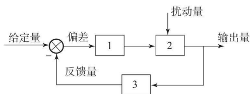
图 1-4 闭环控制系统结构图
