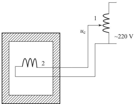
图 1-1 温度控制系统
