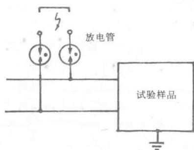
(c) 对称平衡输入（出）有远供电的设备
