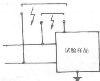
(a) 无远供的设备试验接线
