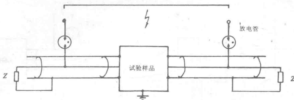
(b) 不对称输入和输出的设备接线
