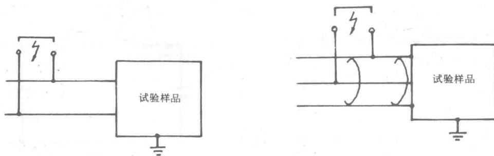
(b) 不对称输入（出）的设备
