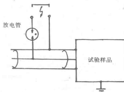
(d) 不对称输入（出）有远供电的设备
