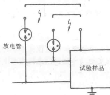
(b) 有远供的设备试验接线
