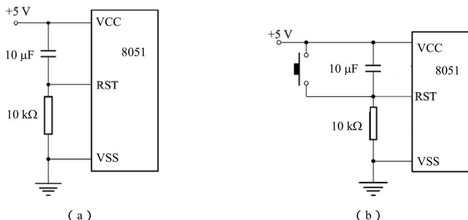
图 1.7 复位电路
