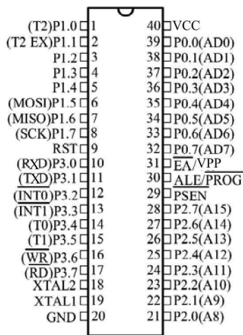
图 1.5 PDIP40 封装的单片机引脚排列
