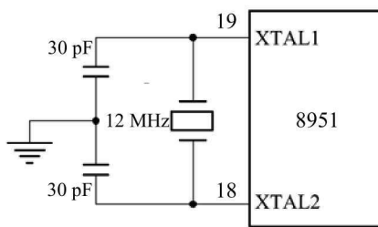
图 1.6 时钟电路
