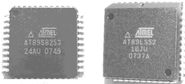
图 1.4 QFP 和 PLCC 封装的单片机
