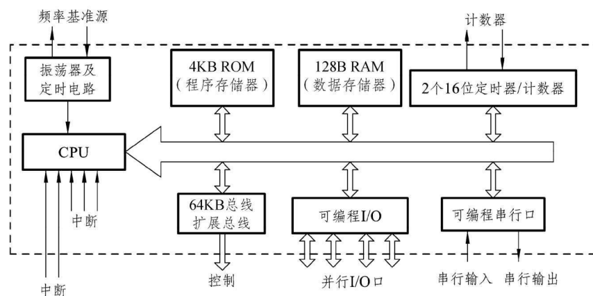
图 1.9 51 单片机的内部基本结构
