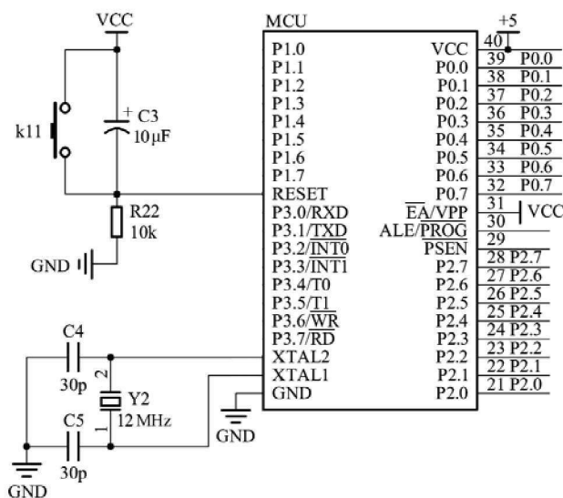
图 1.8 单片机最小系统电路
