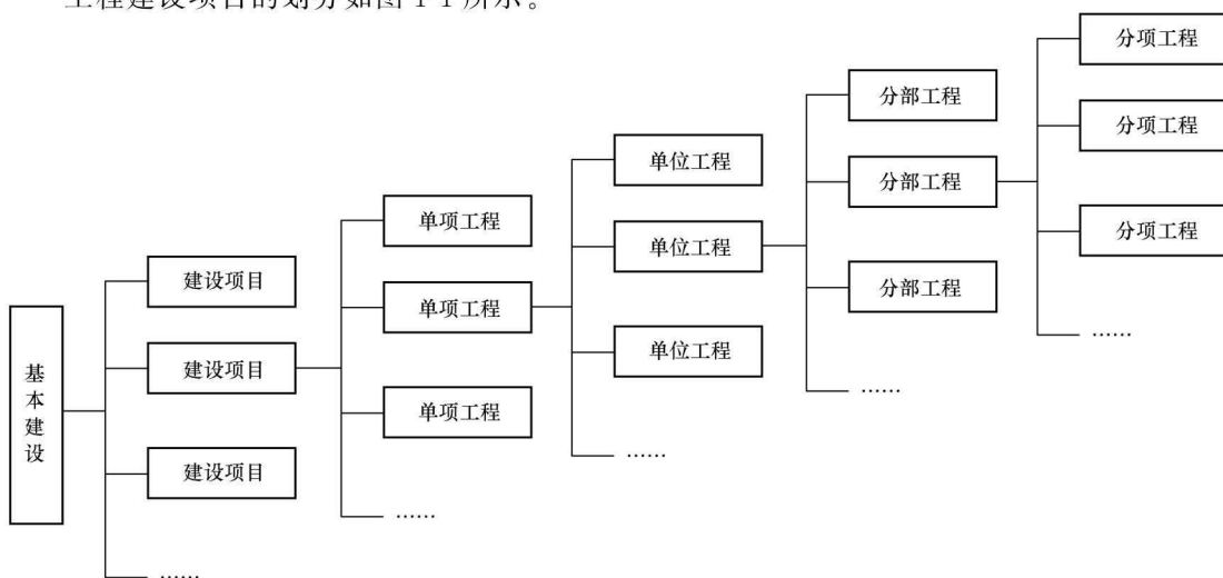
图 1-1 工程建设项目的划分
