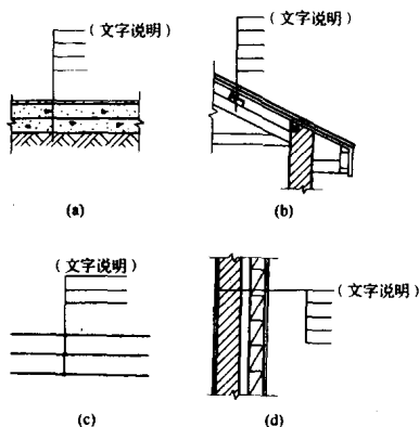
图 6.3.3 多层构造引出线
