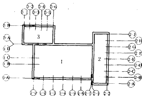
图 7.0.5 定位轴线的分区编号
