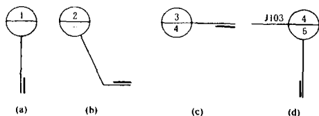
图 6.2.2 用于索引剖面详图的索引符号
