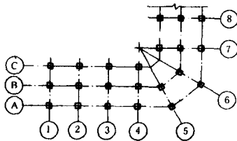
图 7.0.10 折线形平面定位轴线的编号
