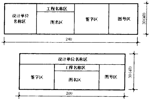
图 2.2.2 标题栏
