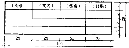
图 2.2.3 会签栏
