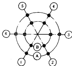
图 7.0.9 圆形平面定位轴线的编号
