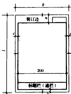
图 2.1.1-3 A4 立式幅面
