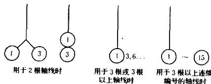
图 7.0.7 详图的轴线编号
