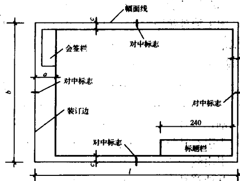
图 2.1.1-1 A0~A3 横式幅面
