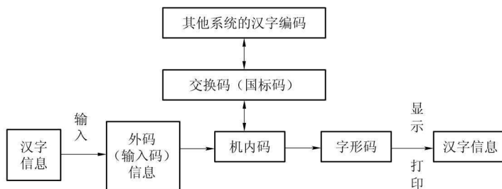
图 1-3 汉字编码之间的关系
