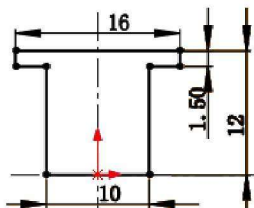
图 1.3 横断面草图 1
